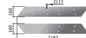
Лемеж двустранен ляв Р33 КГЮ.01.545-01 десен Р33 КГЮ.01.546-01 M (на един)=13,3 кг
