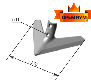
Лапа «Омичка» (270 мм) СКС.01.08.080-02 Алмаз (65г) М=1,1 кг
