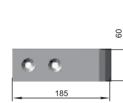
Длето Р33 КША.25.050 M=0,82 кг
