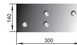
Бокова част (сормайт) Р33.ПЛЖ.51.200-06 М=5,5 кг
