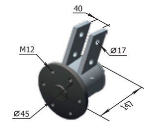
Тяло на лагер Р33.18.14.100 M= 9,43 кг
