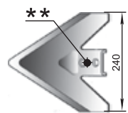
Лапа Salford (240 мм) РЗЗ.240604.00 М=1,84 кг
