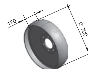
Колело голямо ПНЛ 35.100 M=34 кг
