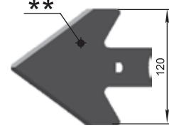
Лапа, която се прикрепя отгоре (120 мм) 61.03.43.004 М=0,34 кг
