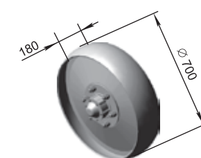
Колело голямо с главина Р33.08.200 M=60 кг
