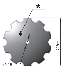
Диск БДМ Р33.1905-22 M=10,97 кг
