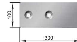
Пълец РЗ3.ПЛЖ.21.500 М=2,3 кг
