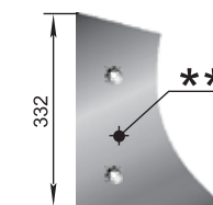
Гръд на отметателна дъска Р33.ПЛЕ.01.401 М=2,0 кг
