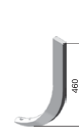
Стълбец КПС Н.043.11.401-03А М=2,63 кг
