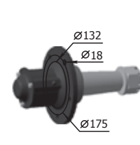
Главина на колело ОС 354.42.03.000-02 М=15,5 кг
