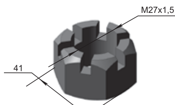
Гайка прорязана 4x4 01.014 M=0,163 кг
