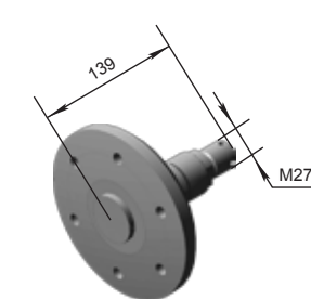
Главина Р33.18.14.103 M=4,43 кг
