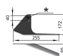
Лапа на бръснач КРН (85 мм) Р33.00.220-04 дясна/ Р33.00.220-05 лява М (на една)=0,71 кг
