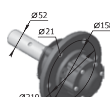
Главина на колело ПНЛ.Р33.16.100 M=23 кг
