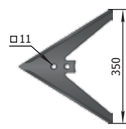
Лапа КШУ-12 Н.043.05.402-02 М=1,37 кг
