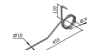
Зъб пружинен десен (КШУ) Р33.КЦД.00.601 М=0,66 кг
