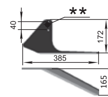
Лапа на бръснач КРН (150) Р33.00.220 дясна/ Р33.00.220-01 лява М=1,3 кг
