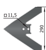
Лапа ДжонДир-290 М=1,4 кг
