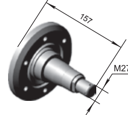
Ос БДМ 4x4 01.103 M=4,55 кг
