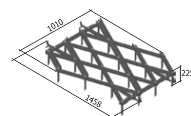
Брана зъбна БЗТ-1.0.00.000-02 M=47 кг
