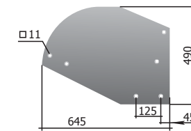
Крило на отметателна дъска Р33.ПНЛ.01.411 М=13,4 кг
