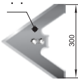
Лапа за сеитба (300 мм) СКС.01.08.080-01 М=1,38 кг
