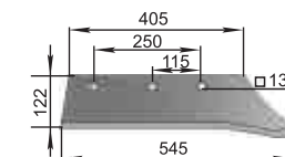
Лемеж ПЛЖ Р33.31-702 Подсилен, 12 мм М=4,9 кг
