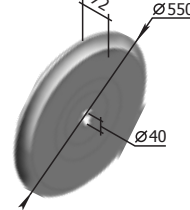
Валяк СЗЮ.00.160 М=13 кг
