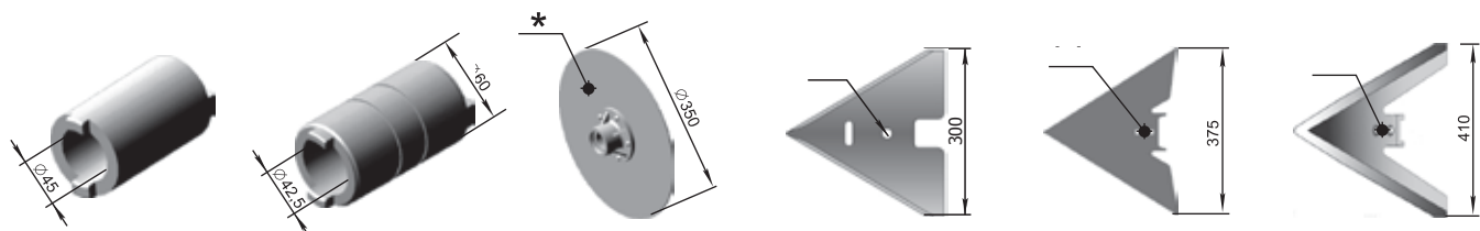
Втулка СЗР.00.800 (за сеялка СЗС-2) М=1,15 кг
