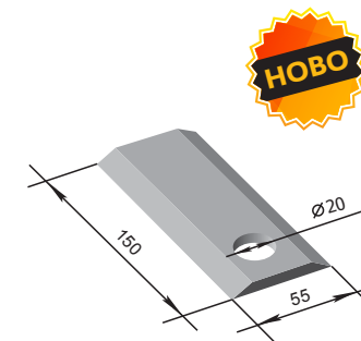
Нож КРН къс РЗЗ.00.151 М=0,3 кг
