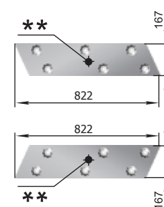
Лемеж двустранен ляв Р33 КГП 01.545В десен Р33 КГП 01.546В M (на един)=8,78 кг
