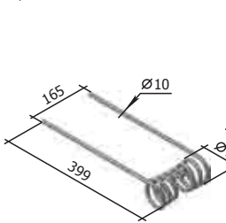
Зъб пружинен към брана Р33.01.601 БЗГ 15, 18, 24 (d=10 мм) M=1,2 кг
