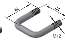
Скоба (М12) КПД.55.00/21 М=0,18 кг
