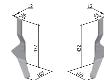
Стълбец събран КРН Н.043.01.100-06 (десен), Н.043.01.100-07 (ляв) М=2,46 кг
