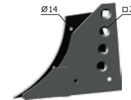
Подложка Р33.ПЛЕ 21.100 (отливане) М=17 кг
