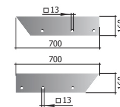
Лемеж ляв Р33.КГЮ.01.545К десен Р33 КГЮ.01.546К M (на един)=8,58 кг
