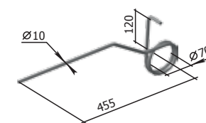
Зъб пружинен ляв (КШУ) Р33.КЦД.00.601-01 М=0,66 кг
