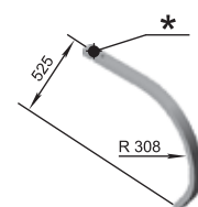
Стилбец РЗЗ.043.13.401-02/01 М=12 кг
