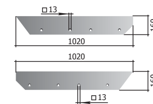
Лемеж ляв Р33.КГЮ.01.545 десен Р33 КГЮ.01.546 M (на един)=13,3 кг
