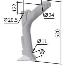
Стилбец СКП 01.08.060 «Омичка» М=5,5 кг
