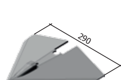
Лапа на ботуш РЗЗ.АУП.18.02.020Г М=1,80 кг
