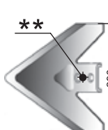
Лапа Salford (290 мм) Р33.290604.00 М=2,07 кг
