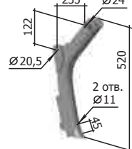
Стилбец СКС 01.08.030 М=4,95 кг
