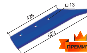
Лемеж АЛМАЗ ПНЧС 01.700 М=4,72 кг
