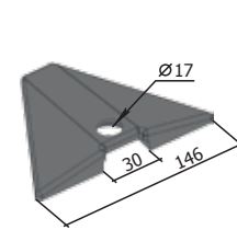
Подложка РЗЗ.АУП.18-03.02.303 М=0,60 кг
