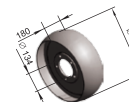
Колело малко ПЛУ 06.500 М=21,1 кг
