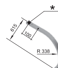
Стълбец Р33.043.13.401 М=13,15 кг
