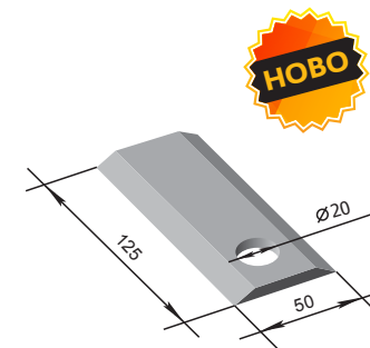
Нож КРН къс РЗЗ.00.125 М=0,2 кг
