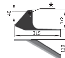
Лапа на бръснач КРН (120 мм) Р33.00.220-02 дясна/ Р33.00.220-03 лява М=0,8 кг
