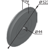
Валяк СЗШ.00.370 М=8,70 кг
