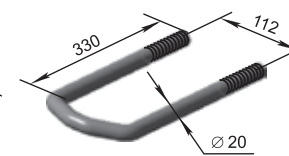
Скоба (М20) КТА.27.601 М=1,86 кг
