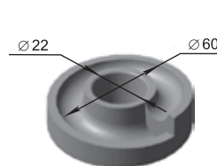
Упор под пружина КТА.27.201 М=0,21 кг
