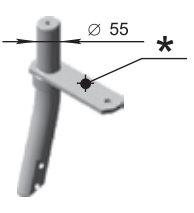
Сълбец на завои на режеш възел (55 мм) 4x4 01.021.00.000 M=10,6 кг
