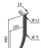
Лапа 8,5 Н.043.08.401-04 М=2,2 кг
