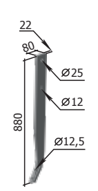
Стълбец АПК. 02.01.000 (22мм) М=10,95 кг
