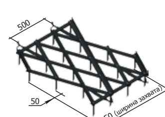
Брана зъбна БЗС-1.00.000 M=34,10 кг
