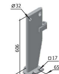
Сълбец КША.25.010 M=26,6 кг
