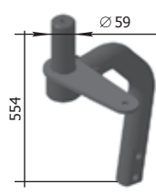
Сълбец за дискова брана с развърнат диск Р33.25.20.100-01 M=18,4 кг
