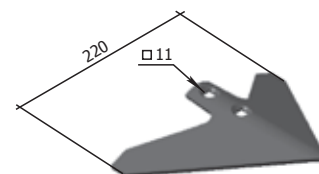
Лапа С-5,1 Н.043.05.110 М=0,77 кг
