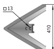
Лапа (410) РЗЗ.043.03.110 М=4,55 кг
