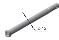
Ос на батерия БДБ 04.613/ БДБ 04.614 L=1450, M=18,1 кг L=1750, M=20,58 кг
