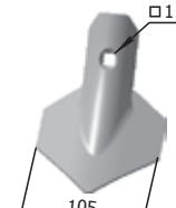
Лапа, която се прикрепя отгоре Европак 61.03.43.004 М=0,34 кг
