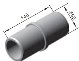
Втулка БДО 01.802-01 M=1,3 кг
