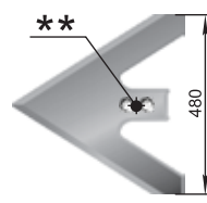
Лапа (480 мм) АПК 7.2 М=4,5 кг
