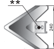
Лапа Salford (240 мм) Р33.240604.00 М=1,84 кг
