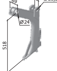
Стилбец СКС 01.08.140 М=8,55 кг
