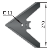
Лапа за сеитба «Омичка» (270 мм) СКС.01.08.080-02 М=1,1 кг
