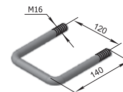
Скоба (М16) КПД.55.00/22 М=0,65 кг
