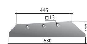
Лемеж Р33.П-01-710 М=6 кг
