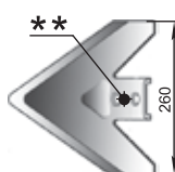
Лапа Salford (260 мм) РЗЗ.260604.00 М=1,91 кг
