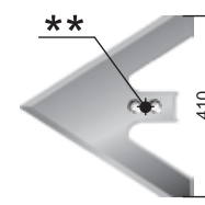
Лапа (410 мм) Р33.043.03.110 М=4,0 кг
