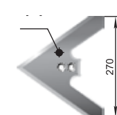
Лапа за сеитба (270 мм) СКС.01.08.080 М=1,17 кг
