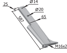
Стилбец РЗЗ.АУП. 18-03.02.010 М=8,10 кг
