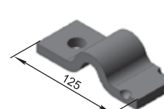
Притискач КТА 27.502 М=0,56 кг
