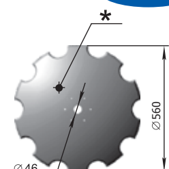
Диск БДМ АМА (560 мм) M=10,9 кг
