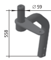
Сълбец за дискова брана с развърнат диск Р33.22.10.200-01 M=15 кг
