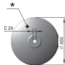
Диск ЛДГ С-1-1-450-5-29 Р33 407.001 M=6,3 кг
