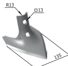
Лапа КБМ-10,8 Р33.00.01.604 М=0,60 кг
