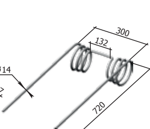
Зъб пружинен Р33.00.01.602 (d=14mm) M= 4 кг
