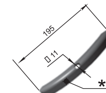
Наралник, който прикрепя отгоре 61.03.43.003 М=0,29 кг
