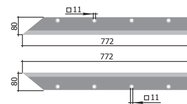
Лемеж ляв Р33 КША 07.030, десен Р33 КША 07.030-01 M (на един)=3,53 кг
