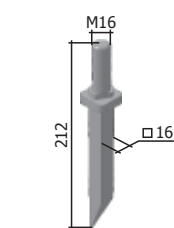
Зъб на брана БЗСС-1 M=0,36 кг
