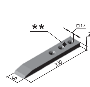
Длето КГЮ 11.300А M=2,8 кг
