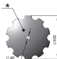
Диск БДТ Р33.428.001 лист-10 (за брани) M=15,5 кг
