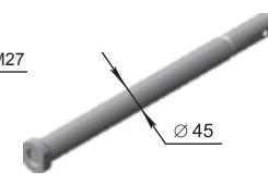
Ос на батерия БДО 01.625/ БДО 16.626 L=1700, M=4,6 кг L=1920, M=23,96 кг
