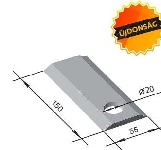
KPH kés rövid P33.00.151 W=0,3 kg
