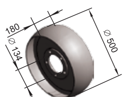
Kis kerék ПЛН 06.500 M=21,1 kg
