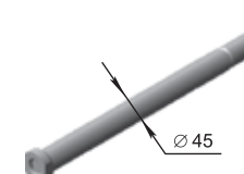
Elem tengelye БДБ 04.613/БДБ 04.614 L=1450, M=18,1 kg L=1750, M=20,58 kg
