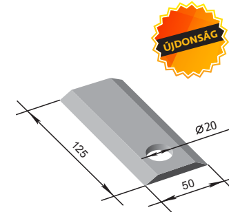
KPH kés rövid P33.00.125 W=0,2 kg
