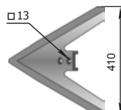
Láb (410 mm) P33.043.03.110 W=4,55 kg
