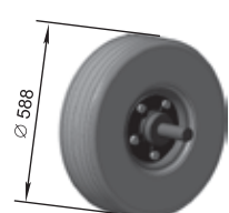
Gumiabroncsos kerék ПЧ-2,5 P33.14.05.700 M=39,5 kg
