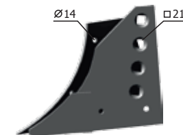
Eketalp P33.ПЛЕ 01.100 (fémjelzett-hegesztett) M=14 kg
