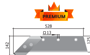
Ekevas egyenes bittel bal P33.11.51.200-02 M=5,51 kg
