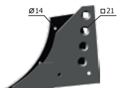
Eketalp P33.ПЛЕ 01.100 (fémjelzett-hegesztett) M=14 kg
