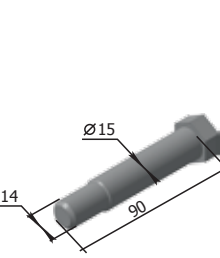
Csavar P33.11.04.104 M=0,15 kg
