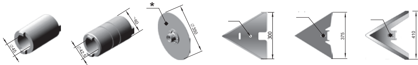
Gyűrű C3P.00.800 (vetőgépre C3C-2) W=1,15 kg
