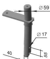
Állvány P33.47.01.100 M=10,9 kg
