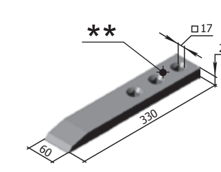
Egyenes szárú bit КГЮ 11.300A M=2,8 kg
