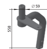
Állvány korongléc számára Kifordított koronggal P33.22.10.200-01 M=15 kg
