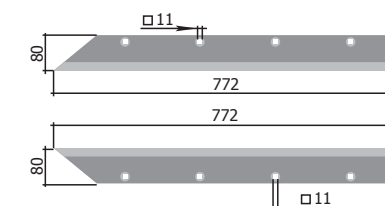
Bal ekevas P33 КША 07.030, jobb P33 КША 07.030-01 M (egy)=3,53 kg
