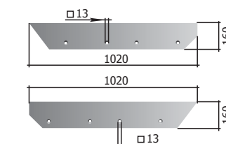
Bal ekevas P33.КГЮ.01.545, jobb P33 КГЮ.01.546 M (egy)=13,3 kg
