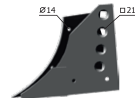
Eketalp P33.ПЛЕ 21.100 (öntött) M=17 kg
