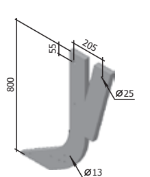
Állvány P33.09.01.100 M=35 kg
