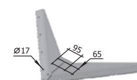
Láb КША.07.070 M=14,7 kg
