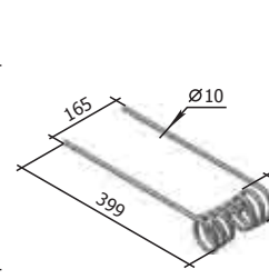
Rugós fog a boronához P33.01.601 Б3Г 15, 18, 24 (d=10 mm) M=1,2 kg
