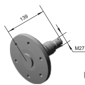
Kerékagy P33.18.14.103 M=4,43 kg
