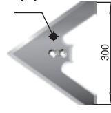
Vetőláb (300 mm) CKC.01.08.080-01 W=1,38 kg
