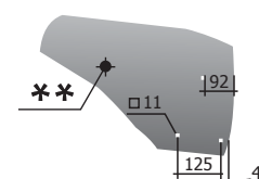
Ekevas szárny P33.ПЛЕ.21.411 M=9,2 kg
