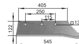
Ekevas ПЛЖ P33.31-702 Erősített, 12 mm M=4,9 kg
