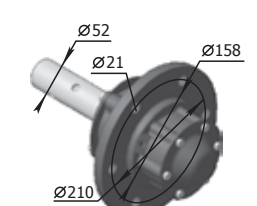
Agykerék ПНЛ.Р33.16.100 M=23 kg
