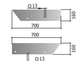
Bal ekevas P33.КГЮ.01.545K, jobb P33 КГЮ.01.546K M (egy)=8,58 kg
