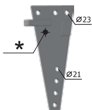
Állvány P33.01.200 (fémjelzett-hegesztett) M=14,3 kg
