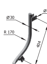
Védőfedél P33.09.01.200 M=3,81 kg
