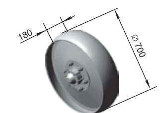
Nagy kerék Kerékaggal P33.08.200 M=60 kg
