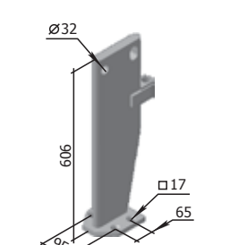
Állvány КША.25.010 M=26,6 kg
