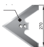
Vetőláb (270 mm) CKC.01.08.080 W=1,17 kg
