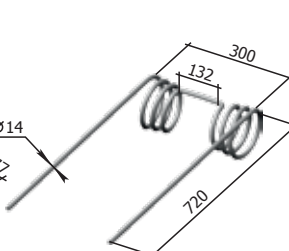
Rugós fog P33.00.01.602 (d=14mm) M=4 kg
