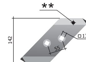
Szerelhető egyenes bit P33.11.51.240 (bal) M=1,36 kg
