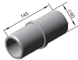
Gyűrű БДО 01.802-01 M=1,3 kg
