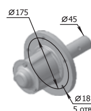
Kerékagy ПЛЕ.Р33.06.200-Б M=13 kg
