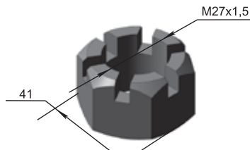
Vésett anyacsavar 4x4 01.014 M=0,163 kg
