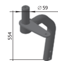
Állvány korongléc számára Kifordított koronggal P33.25.20.100-01 M=18,4 kg
