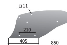
Ekeszegy bal P33.11.51.003-02 M=11,5 kg
