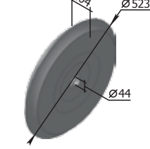
Henger C3W.00.370 W=8,70 кг
