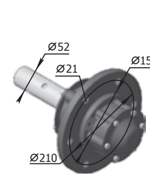
Kerékagy ПНЛ.Р33.16.100 M=23,0 kg
