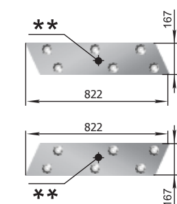
Kétoldalú ekevas bal P33 КГП 01.545B, jobb P33 КГП 01.546B M (egy)=8,78 kg
