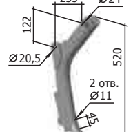
Állvány CKC 01.08.030 W=4,95 kg
