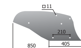
Ekeszegy jobb P33.П.401-02A M=11,5 kg
