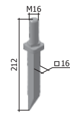
Borona foga Б3СС-1 M=0,36 kg
