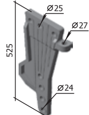
Állvány (öntött) P33.ПЛЕ 31.301 M=17 kg
