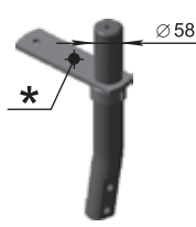
Fordulat állványa vágóegység (58 mm) 4x4 01.022.00.000 M=10,5 kg
