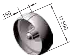
Kis kerék Kerékaggyal P33 06.200 M=35 kg
