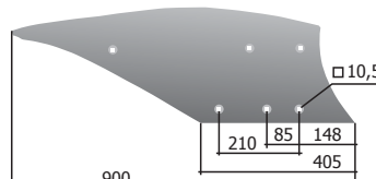
Ekeszegy P33.31.001 M=11,30 kg
