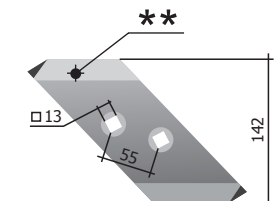
Szerelhető egyenes bit P33.11.31.240 (jobb) M=1,36 kg
