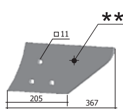
Előke eskeszegye P33.П.402-B M=2,5 kg
