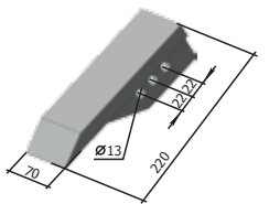
Egyenes bit P33.09.01.300 M=2,9 kg
