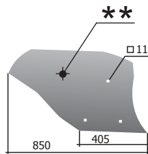
Ekeszegy P33.П.401-A M=11,5 kg
