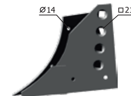
Eketalp P33.ПНЛ 235.01.100 (fémjelzett-hegesztett) M=15,5 kg
