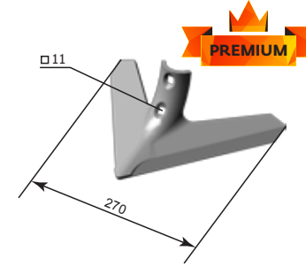
Láb «Omicska» (270 mm) CKC.01.08.080-02 Almaz (65r) W=1,1 kg
