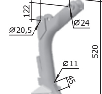
Állvány СКП 01.08.060 «Omicska» W=5,5 kg
