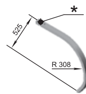
Állvány P33.043.13.401-02/01 W=12 kg
