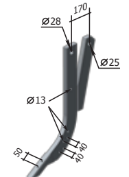
Állvány P33.09.02.600 M=81 kg
