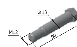
Csavar P33.39.04.102 M=0,12 kg
