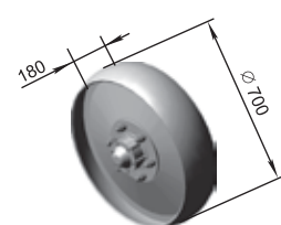
Nagy kerék Kerékgaggal P33 08.200 M=60 kg
