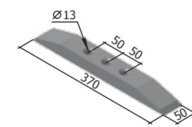
Egyenes bit P33.09.02.310 (kétoldalú) M=5,12 kg
