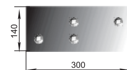
Oldalrész bal P33 11.51.300 jobb P33 ПЛЖ.51.200-06 M (egy)=3,5 kg
