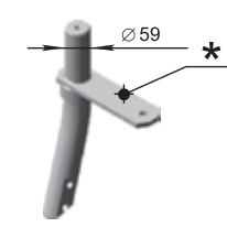
Fordulat állványa vágóegység (59 mm) 4x4 01.021.00.000-01 M=10,8 kg
