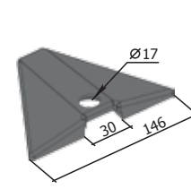
Betét P33.АУП.18-03.02.303 W=0,60 kg
