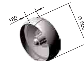
Kis kerék Kerékgaggal P33 06.200 M=35 kg
