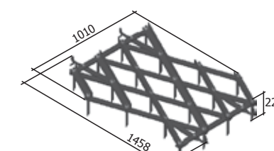
Fogas borona Б3Т-1.0.00.000-02 M=47 kg
