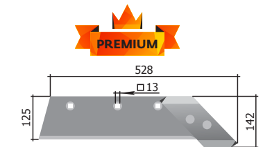
Ekevas egyenes bittel jobb P33.11.31.200-02 M=5,51 kg
