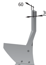
Előke Tartó nélkül P33.02.010 M=11,5 kg
