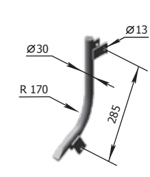
Védőfedél P33.09.01.220 M=3,28 kg
