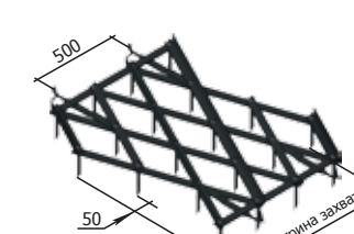
Fogas borona Б3С-1.00.000 M=34,10 kg
