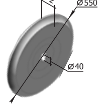
Henger C3W.00.160 W=13 kg
