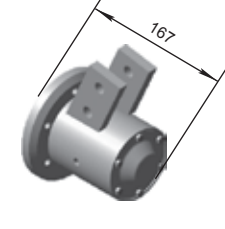
Csapágy BDM váza vágóegység 4x4 01.01.СБ M=11,3 kg
