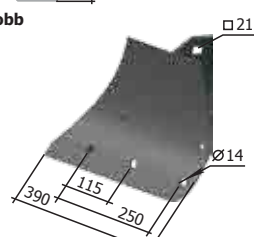
Eketalp bal P33.11.51.100 M=14 kg
