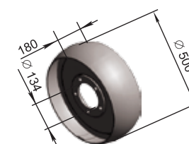
Kis kerék ПЛН 06.500 M=21,1 kg
