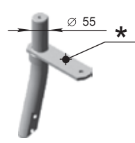
Fordulat állványa vágóegység (55 mm) 4x4 01.021.00.000 M=10,6 kg
