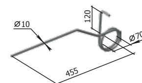
Dinte arcuit stâng (КШУ) P33.КЦД.00.601-01 M=0,66 kg
