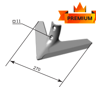
Sapă «Omicika» (270 mm) CKC.01.08.080-02 Almaz (65r) W=1,1 kg
