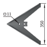
Sapă KШУ-12 H.043.05.402-02 M=1,37 kg
