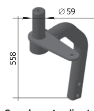
Consola pentru discatori cu disc desfășurat P33.22.10.200-01 M=15 kg
