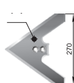
Sapa semănătorii (270 mm) CKC.01.08.080 W=1,17 kg
