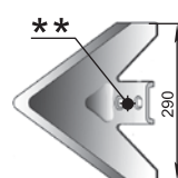
Sapă Salford (290 mm) P33.290604.00 W=2,07 kg
