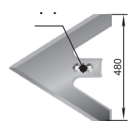
Sapă (480 mm) АПК 7.2 W=4,5 kg
