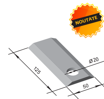
Cuțit KPH scurt P33.00.125 W=0,2 kg
