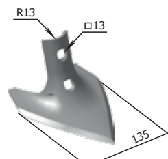
Sapă K5M-10,8 P33.00.01.604 M=0,60 kg
