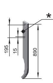
Consolă АПК 01.01.000 (25 mm) M=12 kg
