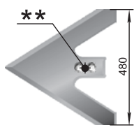
Sapă (480 mm) АПК 7.2 M=4,5 kg
