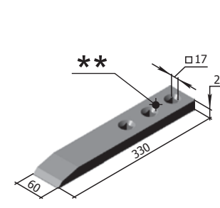
Daltă КГЮ 11.300A M=2,8 kg
