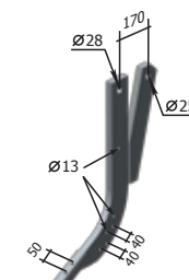
Consolă P33.09.02.600 M=81 kg
