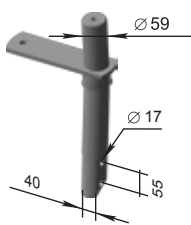
Consolă P33.47.01.100 M=10,9 kg
