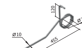
Dinte arcuit drept (КШУ) P33.КЦД.00.601 M=0,66 kg
