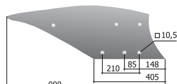
Aripă de rulaj P33.31.001 M=11,30 kg
