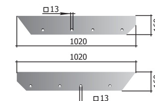
Brăzdar stâng P33.КГЮ.01.545 drept P33 КГЮ.01.546 M (uneia)=13,3 kg
