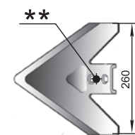
Sapă SALFORD (260 mm) P33.260604.00 M=1,91 kg
