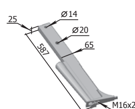
Consolă P33.AYП. 18-03.02.010 W=8,10 kg
