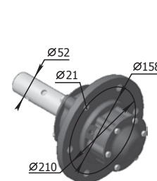
Butucul roții ПНЛ.Р33.16.100 M=23,0 kg
