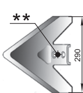
Sapă SALFORD (290 mm) P33.290604.00 M=2,07 kg
