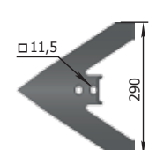
Sapă John Deer-290 M=1,4 kg
