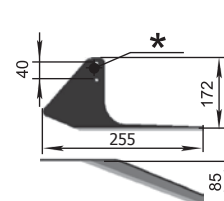
Sapă brici KPH (85 mm) P33.00.220-04 dreapta/ P33.00.220-05 stânga M (egy)=0,71 kg
