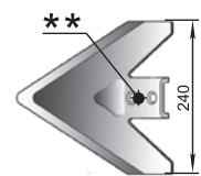
Sapă Salford (240 mm) P33.240604.00 W=1,84 kg
