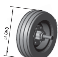
Roată de cauciuc ПЧ-4,5 P33.137.05.000 M=81 kg
