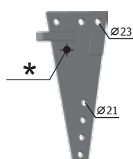
Consolă P33.01.200 (ștanțat-sudată) M=14,3 kg
