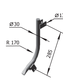
Întăritor P33.09.01.220 M=3,28 kg
