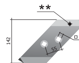
Daltă aplicabilă P33.11.51.240 (stânga) M=1,36 kg
