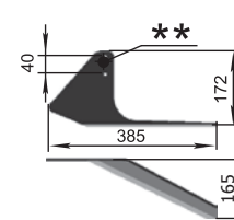
Sapă brici KPH (150) P33.00.220 dreapta/ P33.00.220-01 stânga M=1,3 kg
