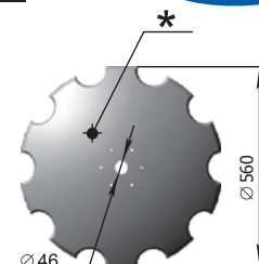
Disc БДМ АМА (560 mm) M=10,9 kg
