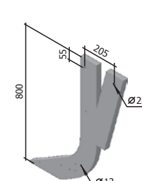
Consolă P33.09.01.100 M=35 kg
