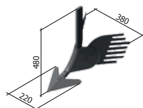
Corp 2H.082.04.000-18 M=8,54 kg
