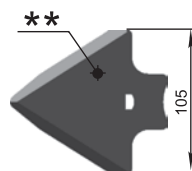
Sapă (105 mm) ART 120 CM-12x4,5 M=0,3 kg
