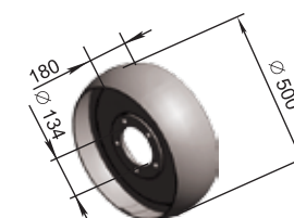
Roată mică ПЛУ 06.500 M=21,1 kg
