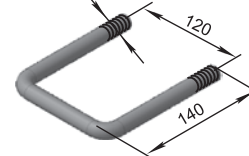
Scoabă (M16) КПД.55.00/22 M=0,65 kg
