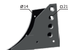
Sabot P33.П/Е 01.100 (ștanțat-sudat) M=14 kg
