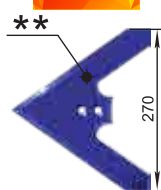
Sapă (270 mm) P33.00.130 ALMAZ M=1,1 kg
