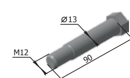
Șurub P33.39.04.102 M=0,12 kg
