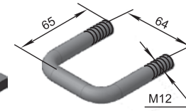
Scoabă (M12) КПД.55.00/21 M=0,18 kg
