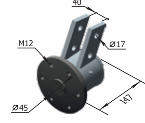
Corpul rulmentului P33.18.14.100 M= 9,43 kg
