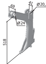
Consolă CKC 01.08.140 W=8,55 kg
