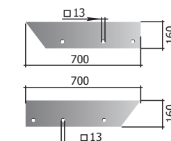
Brăzdar stâng P33.КГЮ.01.545K drept P33 КГЮ.01.546K M (uneia)=8,58 kg
