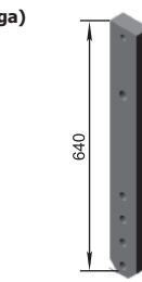
Consolă P33.11.51.006 M=15,3 kg
