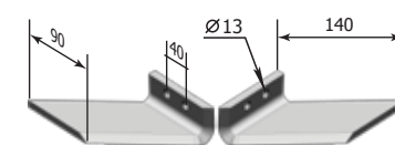
Aripă stângă P33.24.06.120-01 Aripă dreaptă P33.24.06.120 M (uneia)=1,83 kg
