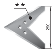
Sapă C4 (290 mm) P33.043.02.110-04 W=1,1 kg
