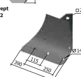
Sabot stâng P33.11.51.100 M=14 kg
