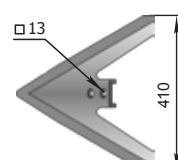
Sapa semănătorii (410 mm) P33.043.03.110 W=4,55 kg
