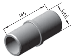
Bucșă БДО 01.802-01 M=1,3 kg
