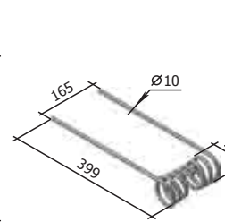
Dinte arcuit pentru grapă P33.01.601 БЗГ 15, 18, 24 (d=10 mm) M=1,2 kg
