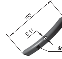
Virf de cuțit aplicabil 61.03.43.003 M=0,29 kg
