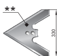
Sapă (330 mm, S=6 mm) P33.00.122 M=1,16 kg
