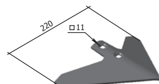
Sapă C-5,1 H.043.05.110 M=0,77 kg
