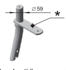
Consola rotirii a nodului de tăiere (59 mm) 4x4 01.021.00.000-01 M=10,8 kg
