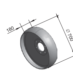
Roată mare ПНЛ 35.100 M=34 kg
