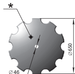
Disc БДТ P33.428.001 lap-10 (на бороны) M=15,5 kg
