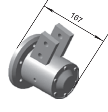
Corpul rulmentului БДМ a nodului tăietor 4x4 01.01.C5 M=11,3 kg
