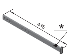
Bară de reglare КПС КЦД-00.412 M=0,86 kg
