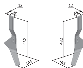
Consolă ansamblată KPH H.043.01.100-06 (dreapta), H.043.01.100-07 (stânga) M=2,46 kg
