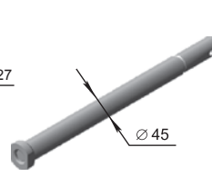
Axa bateriei БДО 01.625/ БДО 16.626 L=1700, M=4,6 kg L=1920, M=23,96 kg
