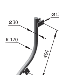
Întăritor P33.09.01.200 M=3,81 kg
