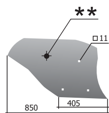
Aripă de rulaj P33.П.401-A M=11,5 kg
