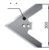
Sapa semănătorii (300 mm) CKC.01.08.080-01 W=1,38 kg
