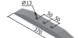
Daltă bit P33.09.02.310 (bilaterală) M=5,12 kg
