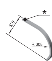
Consolă P33.043.13.401-02/01 W=12 kg
