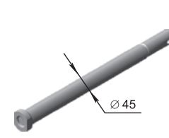
Axa bateriei БДБ 04.613/ БДБ 04.614 L=1450, M=18,1 kg L=1750, M=20,58 kg
