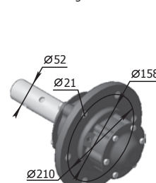
Butucul roții ПНЛ.П33.16.100 M=23 kg
