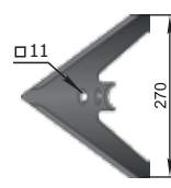
Sapa semănătorii «Omicika» (270 mm) CKC.01.08.080-02 W=1,1 kg
