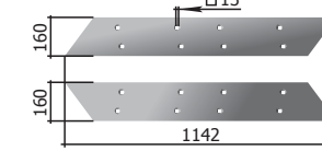
Brăzdar bilateral stâng P33 КГЮ.01.545-01 drept P33 КГЮ.01.546-01 M (uneia)=13,3 kg
