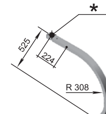
Consolă P33.043.13.401-02/01 M=12 kg
