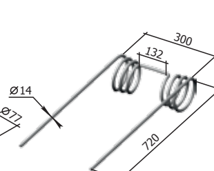
Dinte arcuit P33.00.01.602 (d=14mm) M=4 kg
