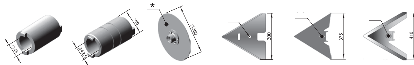
Bucșă C3P.00.800 (pe semănătoarea C3C-2) W=1,15 kg
