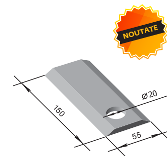
Cuțit KPH scurt P33.00.151 W=0,3 kg
