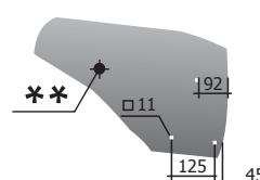
Aripă de rula P33.ПЛЕ.21.411 M=9,2 kg
