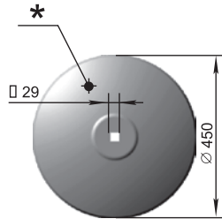
Disc ЛДГ C-1-1-450-5-29 P33 407.001 M=6,3 kg
