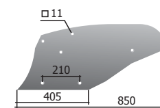
Aripă de rulaj stânga P33.11.51.003-02 M=11,5 kg
