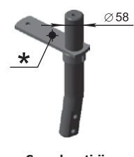
Consola rotirii a nodului de tăiere (58 mm) 4x4 01.022.00.000-01 4x4 01.022.00.000 M=10,5 kg
