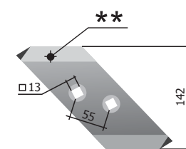
Daltă aplicabilă P33.11.31.240 (dreapta) M=1,36 kg
