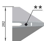
Sapă CKП.03401 (stelth) W=2,1 kg
