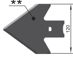
Sapă aplicabilă (120 mm) 61.03.43.004 M=0,34 kg
