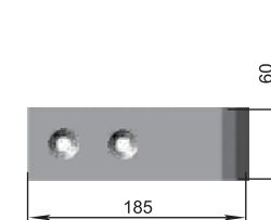
Daltă P33 KWA.25.050 M=0,82 kg
