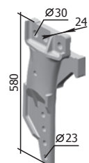
Consolă (turnată) P33.ПНЛ 01.304 M=28 kg
