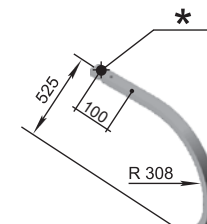
Consolă P33.043.13.401-01 M=12 kg
