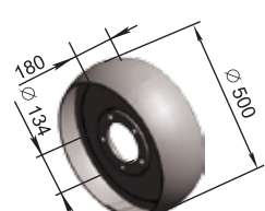
Roată mică ПЛУ 06.500 M=21,1 kg
