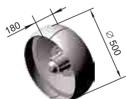
Roată mică cu butuc P33 06.200 M=35 kg
