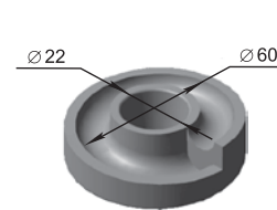
Suport sub arc КТА.27.201 M=0,21 kg
