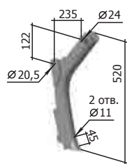
Consolă CKC 01.08.030 W=4,95 kg
