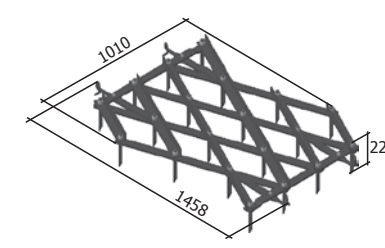
Grăpă cu dinți БЗТ-1.0.00.000-02 M=47 kg
