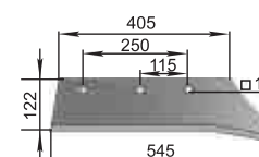
Brăzdar ПЛЖ P33.31-702 Întărit, 12 mm M=4,9 kg
