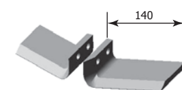
Aripă stângă P33.09.01.400-01 Aripă dreaptă P33.09.01.400 M (uneia)=1,4 kg
