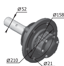
Butucul roții ПНЛ.Р33.16.100 M=23,0 kg
