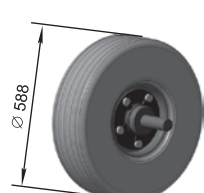
Roată de cauciuc ПЧ-2,5 P33.14.05.700 M=39,5 kg
