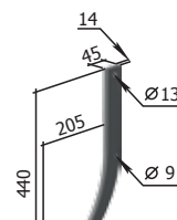
Sapă 8,5 H.043.08.401-04 M=2,2 kg
