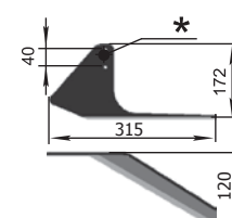
Sapă brici KPH (120 mm) P33.00.220-02 dreapta/ P33.00.220-03 stânga M=0,8 kg
