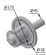
Butucul roții ПЛЕ.Р33.06.200-Б M=13 kg
