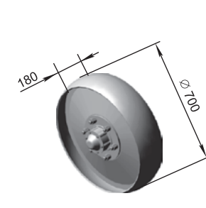
Roată mare cu butuc ПНЛ.П33.16.100 M=60 kg
