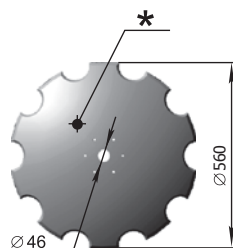
Disc БДМ P33.1905-22 M=10,97 kg
