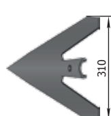
Sapă Bourgault P33.00.310 M=2,53 kg
