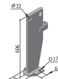
Consolă КWA.25.010 M=26,6 kg
