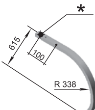
Consolă P33.043.13.401 M=13,15 kg
