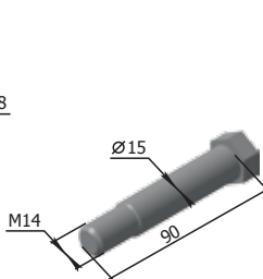
Șurub P33.11.04.104 M=0,15 kg
