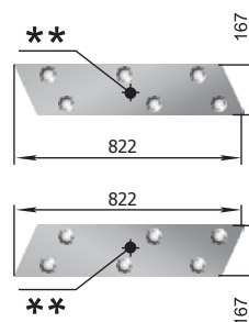
Brăzdar bilateral stâng P33 КГП 01.545B drept P33 КГП 01.546B M (uneia)=8,78 kg
