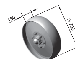
Roată mare cu butuc P33 08.200 M=60 kg
