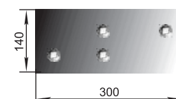
Laterală (sormait) P33.ПЛЖ.51.200-06 M=5,5 kg
