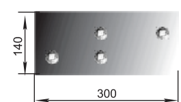
Laterală P33 11.51.300 stânga P33 ПЛЖ.51.200-06 M (uneia)=3,5 kg
