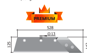
Brăzdar cu daltă drept P33.11.31.200-02 M=5,51 kg
