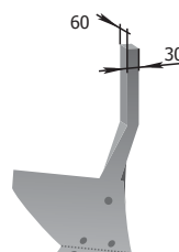
Anibrăzdar fără portsculă P33.02.010 M=11,5 kg
