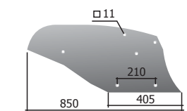
Aripă de rulaj dreapta P33.П.401-02A M=11,5 kg
