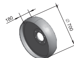
Roată mare ПНЛ 35.100 M=34 kg
