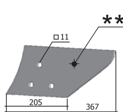
Aripă de rulaj antibrăzdar P33.П.402-B M=2,5 kg
