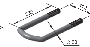
Scoabă (M20) КТА.27.601 M=1,86 kg
