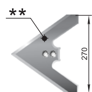
Sapă (270 mm) P33.00.130 M=1,1 kg
