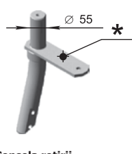
Consola rotirii a nodului de tăiere (55 mm) 4x4 01.021.00.000 M=10,6 kg
