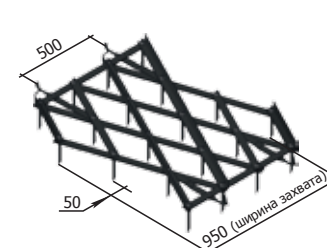
Grăpă cu dinți БЗС-1.00.000 M=34,10 kg
