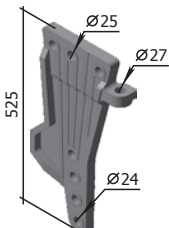
Consolă (turnată) P33.ПЛЕ 31.301 M=17 kg
