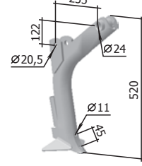
Consolă CKП 01.08.060 «Omicika» W=5,5 kg
