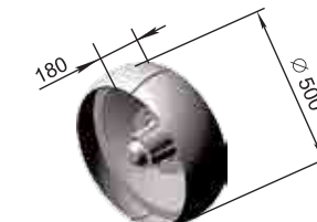
Roată mică cu butuc P33 06.200 M=35 kg
