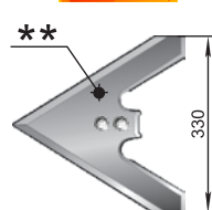
Sapă (330 mm, S=8 mm) P33.00.122-01 M=1,53 kg
